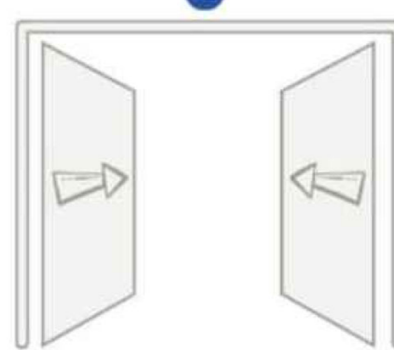
CMB2016
