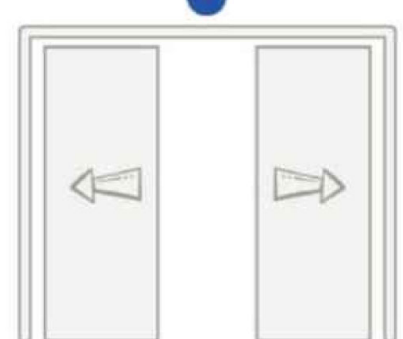
CMB2018
